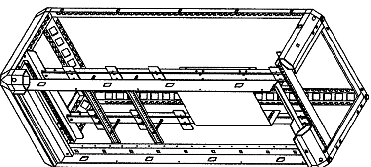
4° MONTAGGIO COPPIA SUPPORTI PANNELLI FRONTALI, CHIUSURE SOPRA E SOTTO 50 mm.
