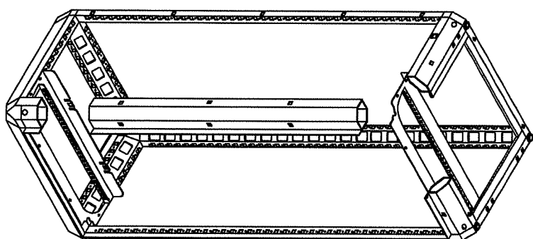
1° MONTAGGIO COPPIA SOSTEGNI ORIZZONTALI INTERNI
