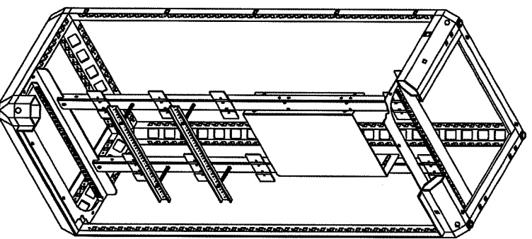
MONTAGGIO PANNELLI INTERNI REGOLABILI PER INTERRUTTORI SCATOLATI, SUPPORTI PER CANALE, RIALZI E GUIDE PER INTERRUTTORI MODULARI.
